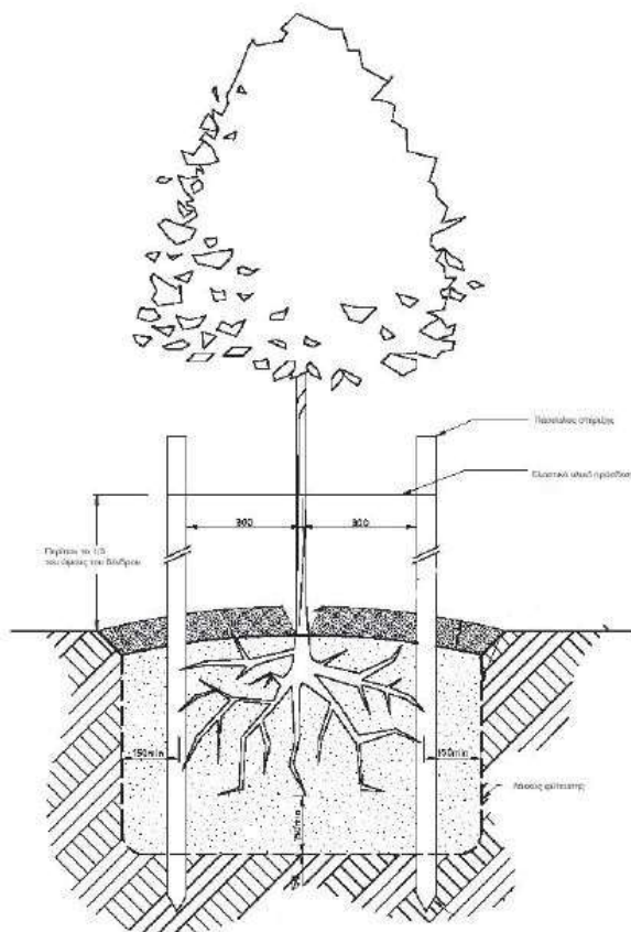
Στήριξη με δύο κατακόρυφους πασσάλους.
